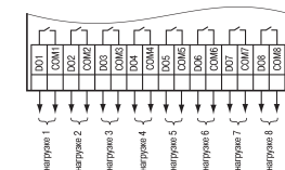
Рисунок 4 – Схема подключения нагрузок к ВЭ типа «Р»
