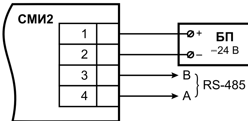
Рисунок 5.1 – Схема подключения
