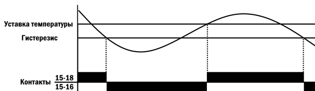
Рис. 3 – Нагрев
