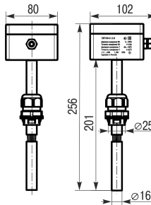
Рисунок 1 – Габаритные и установочные размеры исполнения K1
