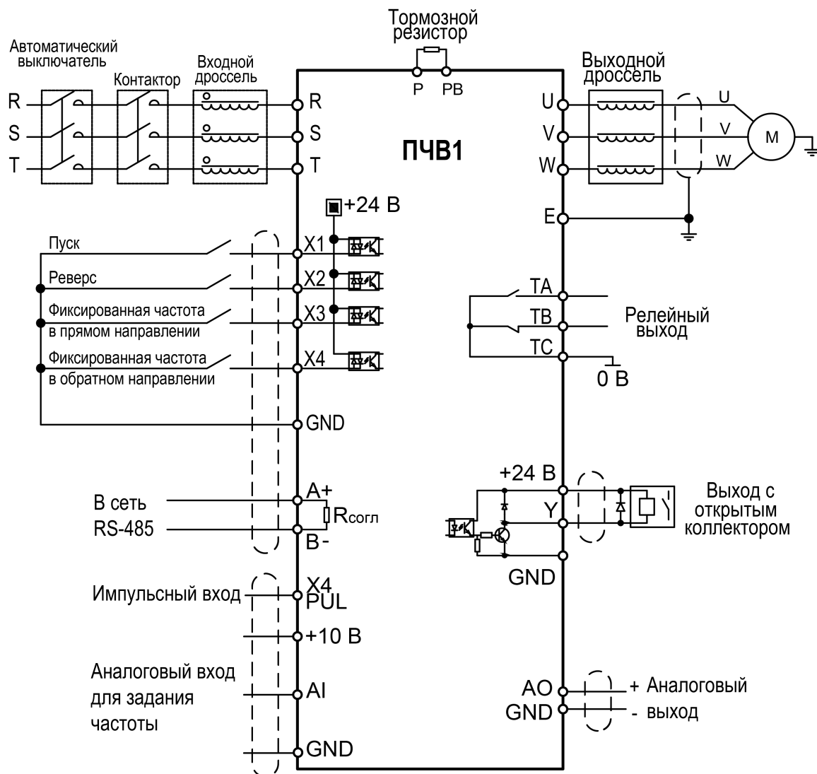
Рисунок 6.5 – Общая схема подключения
