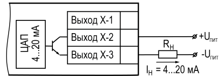
Рисунок 5.21 – Подключение к ВУ типа «И»
