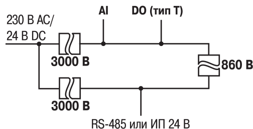
Рисунок 5.2 – Схема гальванической развязки (выход типа «Т»)
