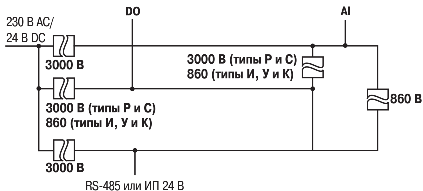
Рисунок 5.3 – Схема гальванической развязки (выходы кроме типа «Т»)
