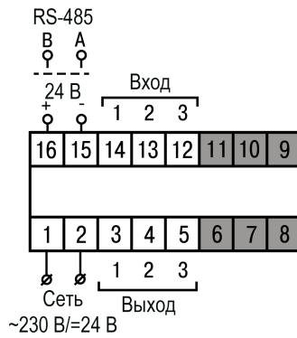
Рисунок 5.5 – Общая схема подключения ТРМ1–Ц5
