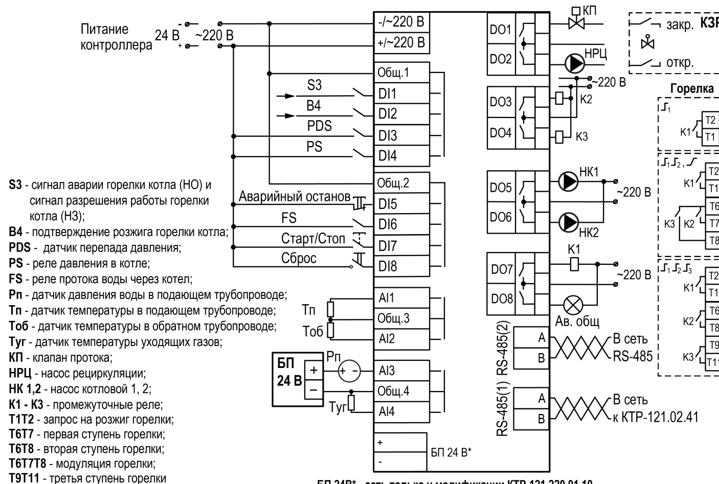
Рисунок 7.4 – Схема подключения
