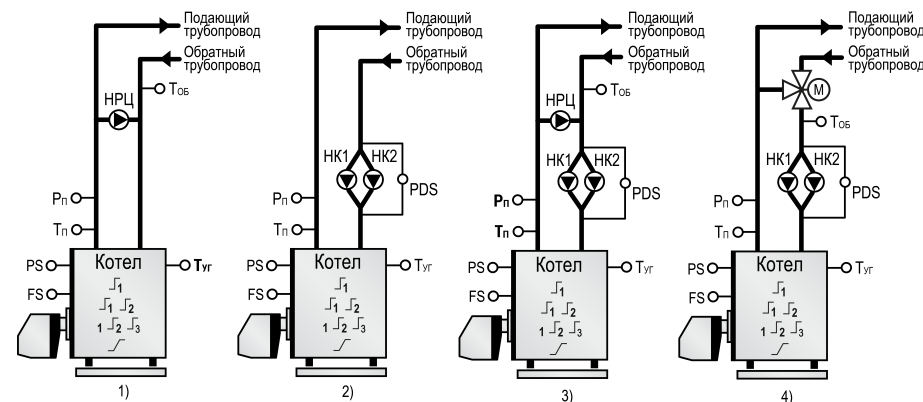
Рисунок 1.1 – Объект управления
