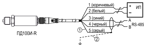
Рисунок 5 – Схема подключения
