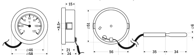
Рис. 3 ART-02 (0...+120°C)
