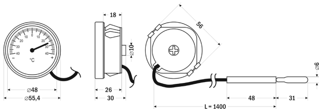
Рис. 2 ART-02 (-40...+40°C)
