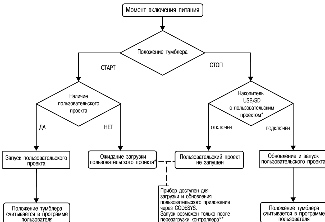
Рисунок 3.8 – Принцип работы тумблера
