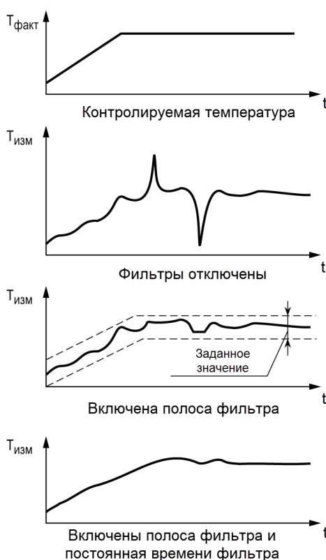
Рисунок 5.23 – Временные диаграммы работы цифровых фильтров
