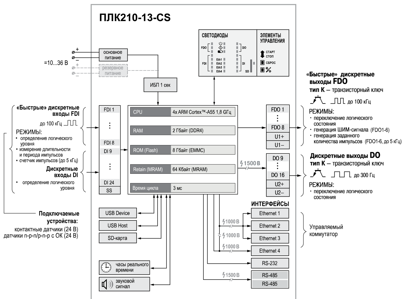
Рисунок 3.3 – Функциональная схема ПЛК210-13-CS
