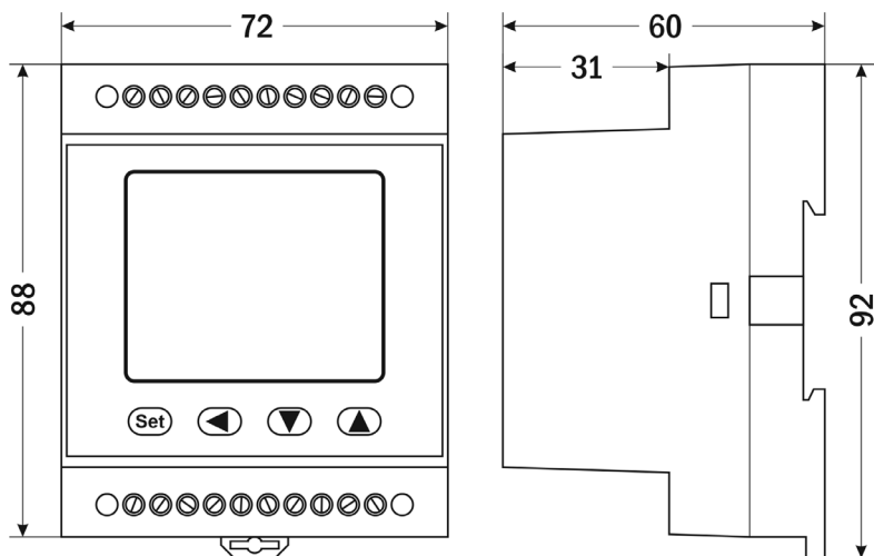
Рис. 2 – Размеры прибора
