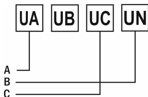
Рис. 6 – Подключение напряжения напрямую до 380 В (трехфазная цепь без нейтрали)
