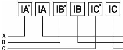
Рис. 8 – Подключение тока напрямую до 5 А
