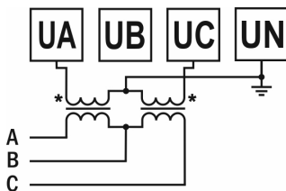
Рис. 7 – Подключение трансформатора напряжения x/380 В (трехфазная цепь без нейтрали)
