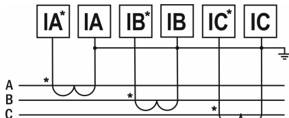
Рис. 9 – Подключение трансформатора тока x/5 А
