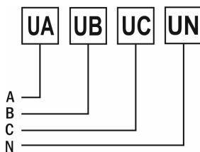
Рис. 4 – Подключение напряжения напрямую до 380 В (трехфазная цепь с нейтралью)
