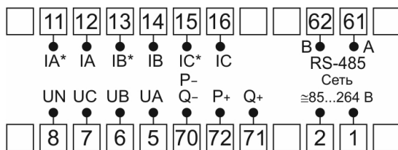
Рис. 3 – Схема подключения
