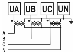
Рис. 5 – Подключение трансформатора напряжения х/380 В (трехфазная цепь с нейтралью)
