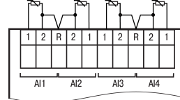
Рисунок 6 – Подключение ТС к AI ПРМ-х.3
