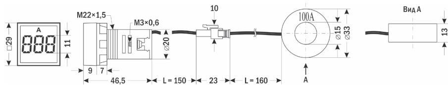
Рис. 7 – Размеры Omix T33-A1-1
