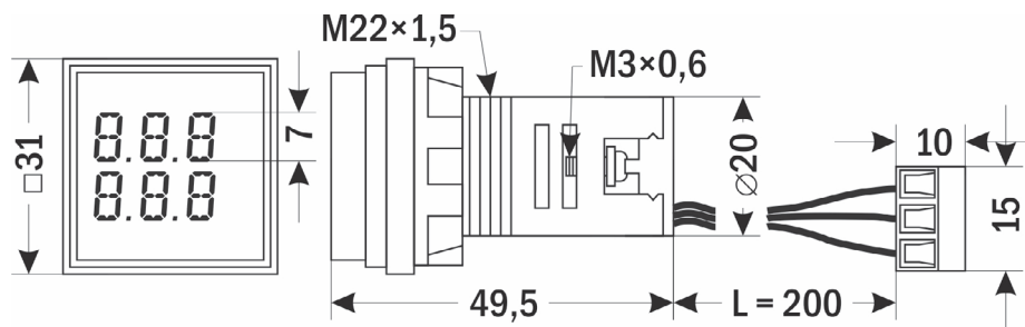
Рис. 7 – Размеры ARCOM T33-HM
