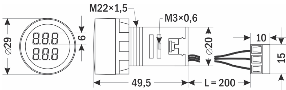
Рис. 6 – Размеры ARCOM R30-HM
