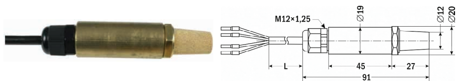
Рис. 7 – Датчик температуры и влажности ARHT-13C
