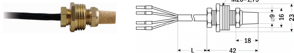
Рис. 6 – Датчик температуры и влажности ARHT-04C
