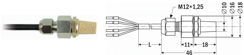
Рис. 4 – Датчик температуры и влажности ARHT-02C
