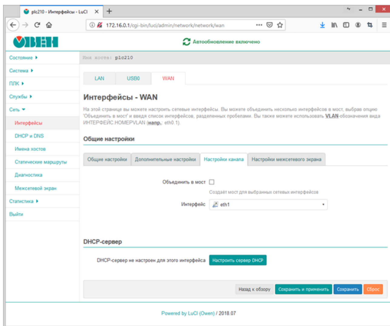
Рисунок 8.12 – Вкладка настроек DHCP-сервера
