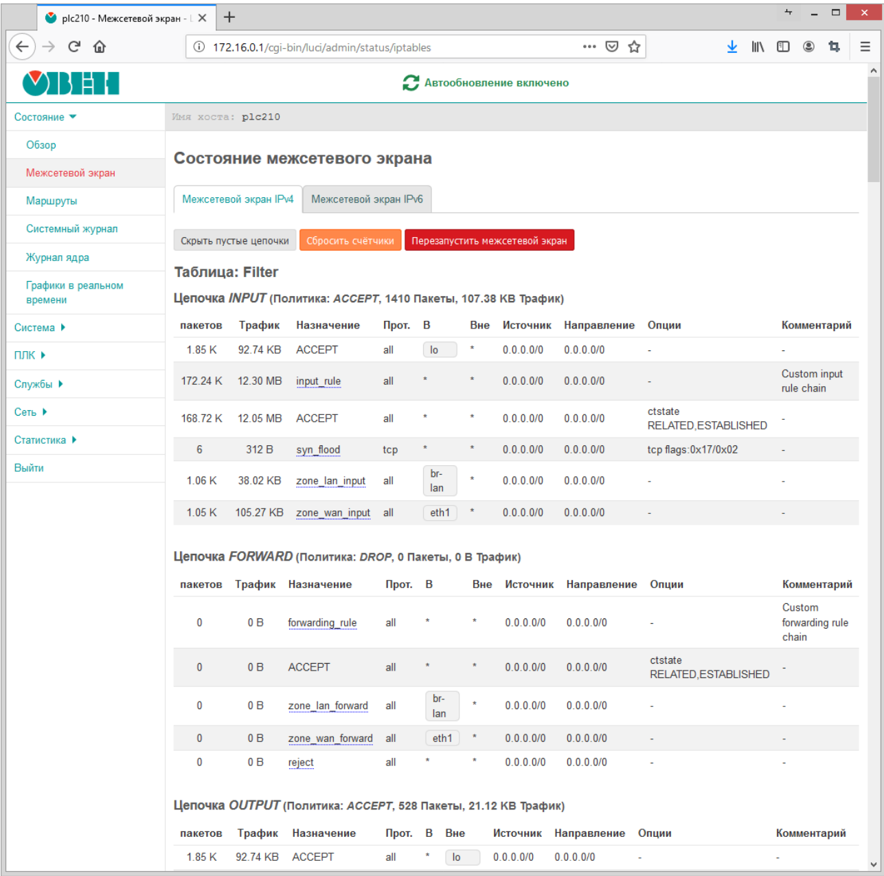
Рисунок 3.12 – Страница «Межсетевой экран»
