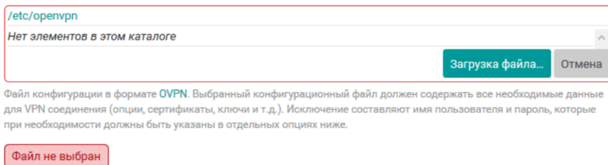
Рисунок 7.40 – Выбор и загрузка конфигурационного файла в формате OVPN. Отсутствие загруженных файлов
