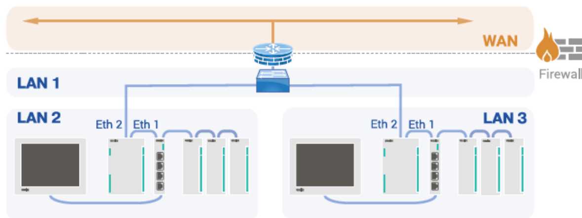
Рисунок 2.10 – Схема №3 сетевых портов контроллера ПЛК200
