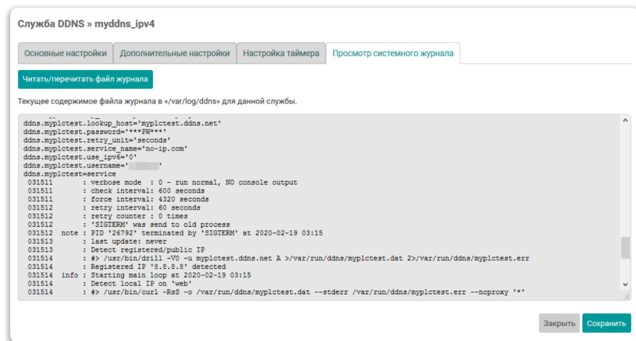
Рисунок 7.17 – Вкладка «Просмотр системного журнала» страницы редактирования DDNS-записи
