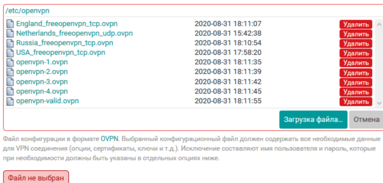
Рисунок 7.39 – Выбор и загрузка конфигурационного файла в формате OVPN. Список загруженных файлов
