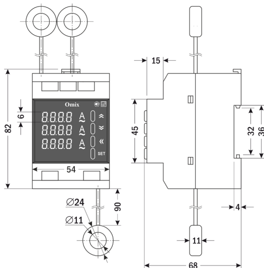
Рис. 2 – Размеры прибора
