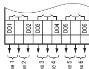
Рисунок 10 – Схема подключения ВЭ типа «Р»
