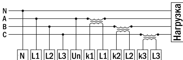
Рис. 3 – Схема подключения
