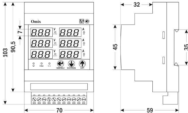
Рис. 2 – Размеры прибора
