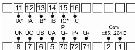
Рис. 3 – Схема подключения D4-M3-3
