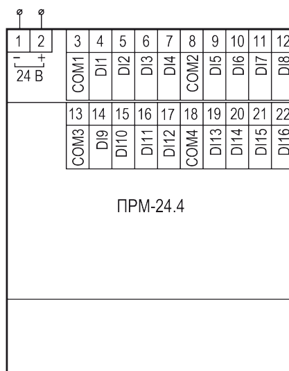
Рисунок 5.2 – Назначение контактов клеммника прибора с питанием 24 В
