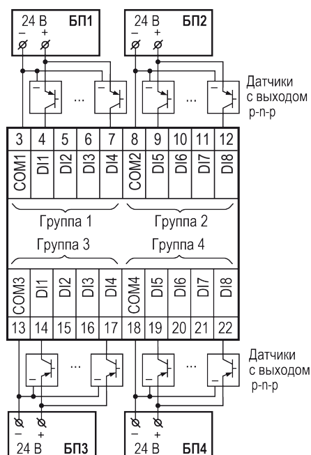
Рисунок 5.8 – Схема подключения датчиков с выходным транзистором р-п-р-типа
