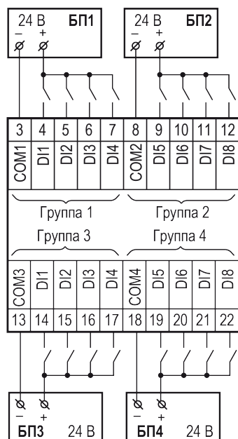
Рисунок 5.6 – Схема подключения дискретных датчиков с питанием 24 В
