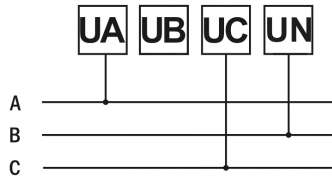
Рис. 10 – Подключение напрямую. Трехфазная цепь без нейтрали (если U \leq 500 В)
