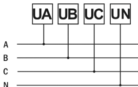
Рис. 9 – Подключение напрямую. Трехфазная цепь с нейтралью (если U \leq 500 В)
