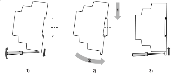
Рисунок 1 – Монтаж прибора
