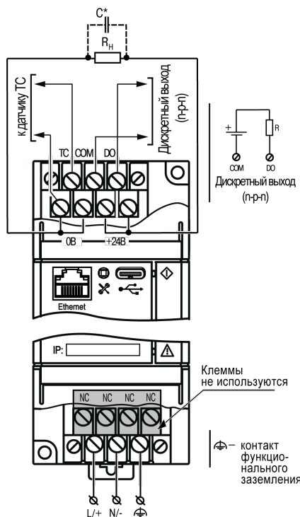
Рисунок 5.1 – Схема подключения прибора
