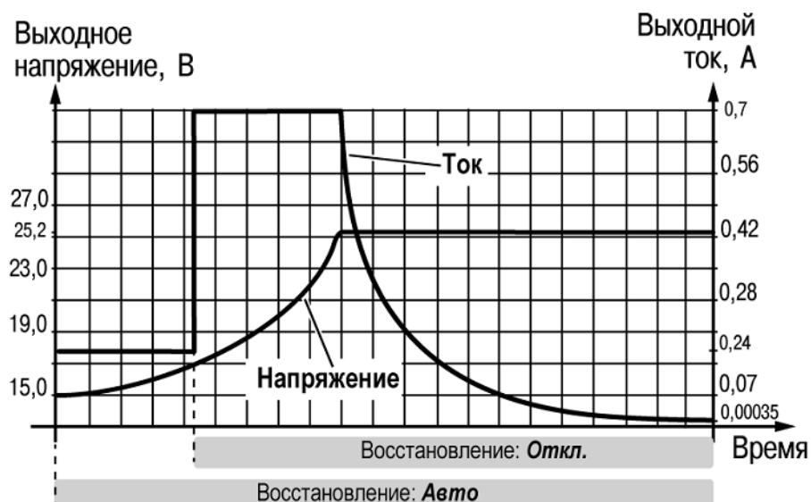
Рисунок 6.1 – График заряда Li-ion АКБ (на примере БА24-2,4) в режиме Авто
