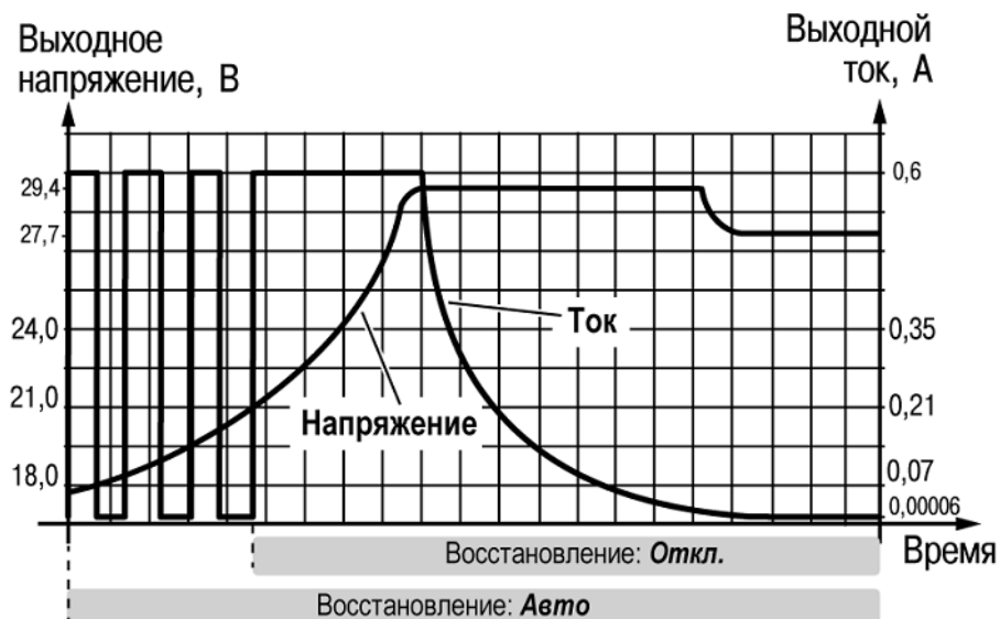
Рисунок 6.2 – График заряда АКБ типа Pb (на примере Pb 2,2) в режиме Авто
