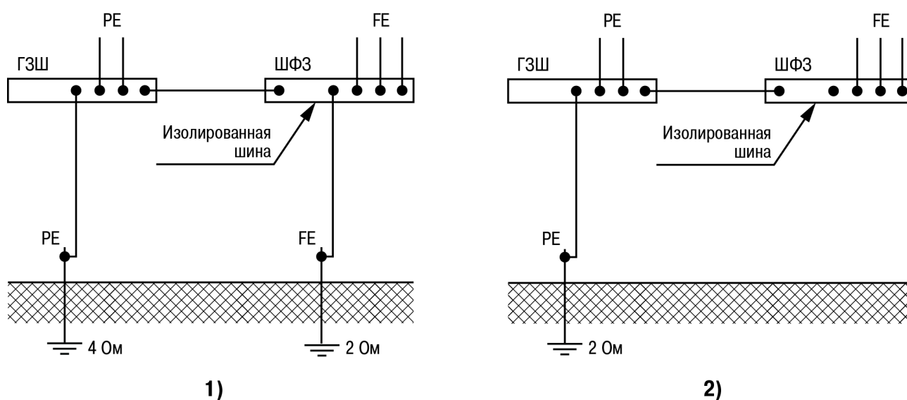
Рисунок 5.3 – Схемы функционального заземления
