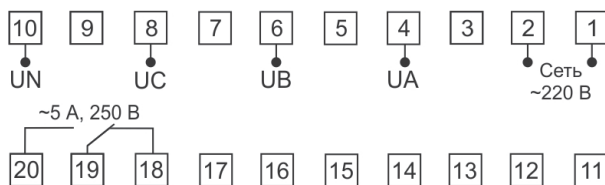
Рис. 4 – Клеммы подключения
