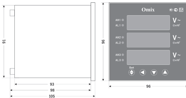
Рис. 3 – Размеры прибора
