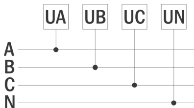
Рис. 5 – Схема подключения
