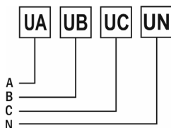
Рис. 5 – Подключение напряжения напрямую (трехфазная цепь с нейтралью)
