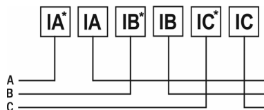
Рис. 6 – Подключение тока напрямую
