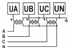
Рис. 8 – Подключение трансформатора напряжения (трехфазная цепь с нейтралью)
