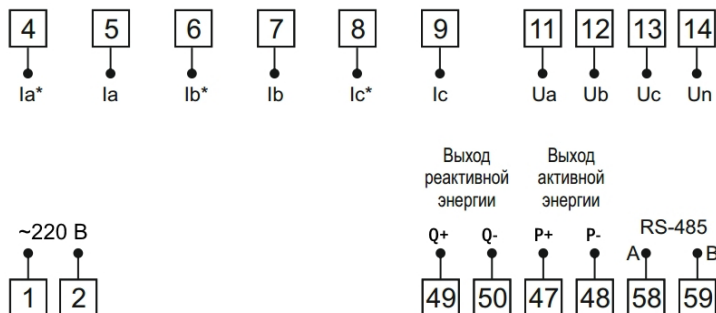
Рис. 3– Схема подключения
