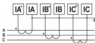
Рис. 9 – Подключение трансформатора тока
