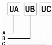
Рис. 4 – Подключение напряжения напрямую (трехфазная цепь без нейтрали)
