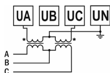
Рис. 7 – Подключение трансформатора напряжения (трехфазная цепь без нейтрали)
