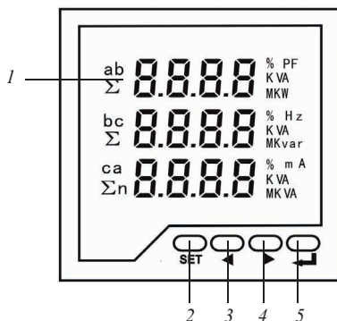
Рис. 1 – Управляющие элементы
