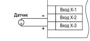
Рисунок 10 – Схема подключения активного датчика с выходом в виде напряжения −50...+50 мВ или 0...1 В
