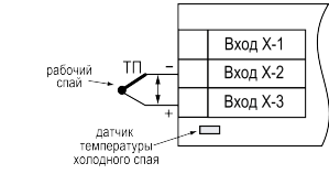
Рисунок 8 – Схема подключения термопары
