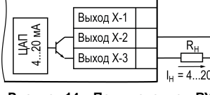
Рисунок 14 – Подключение к ВУ типа «И»
