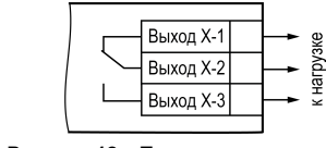
Рисунок 12 – Подключение нагрузки к ВУ типа «Р»
