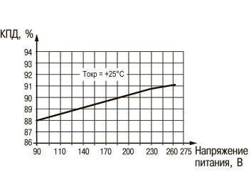
Рисунок 9 – График зависимости КПД от напряжения питания
