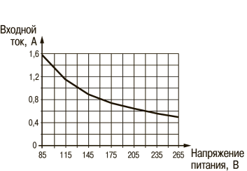
Рисунок 7 – График зависимости входного тока от напряжения питания (Uвых = 24 В, режим Стенд)
