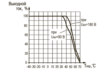
Рисунок 8 – График зависимости выходного тока (Iвых = 24 В, режим Стенд) от температуры окружающей среды (дерейтинг)
