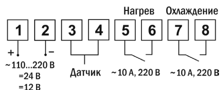
Рис. 3 – Схема подключения
