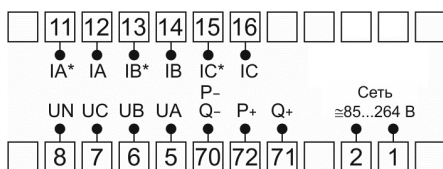
Рис. 3 – Схема подключения D4-MY-3
