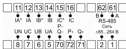
Рис. 4 – Схема подключения D4-MY-3-RS485
