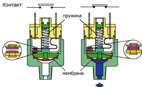
Рис. 1 – Принцип действия
