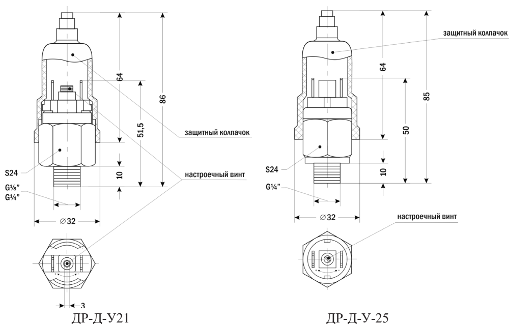
Рис. 9 – Размеры приборов
