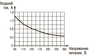
Рисунок 7 – График зависимости входного тока от напряжения питания (Uвых = 12 В, режим Стенд)
