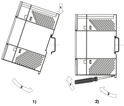
Рисунок 4 – Монтаж (1) и демонтаж (2) прибора
