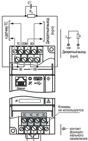
Рисунок 5 – Схема подключения
