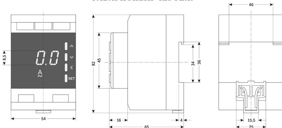
Рис. 2 – Размеры прибора
