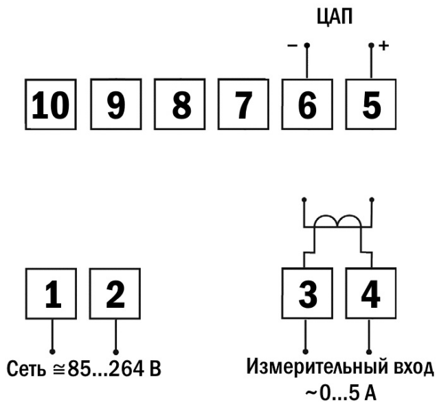
Рис. 3 – Схема подключения прибора.
