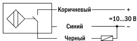
AR-LM6-3001PA PNP
