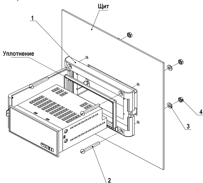
Рисунок 1 – Монтаж в щит прибора в корпусе Щ2
