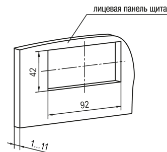
Рисунок 2 – Монтажный вырез под прибор в корпусе Щ2
