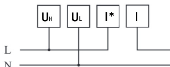
Рис. 6 – Подключение напрямую
