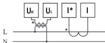
Рис. 7 – Подключение трансформаторов и напряжения
