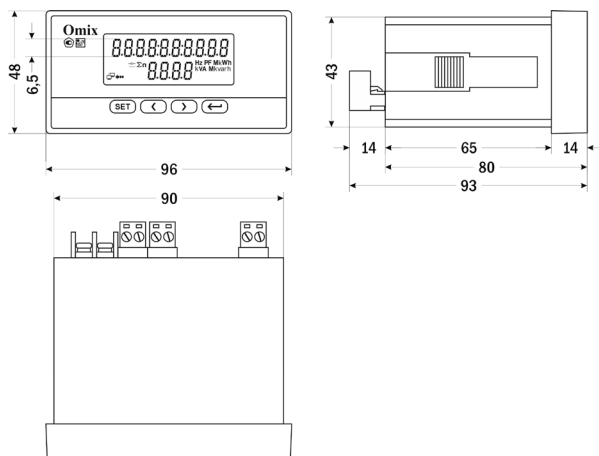
Рис. 4 – Размеры прибора
