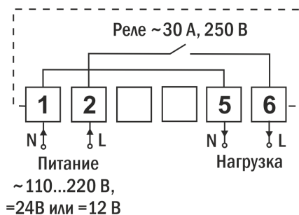
Рис. 4 – Схема подключения
