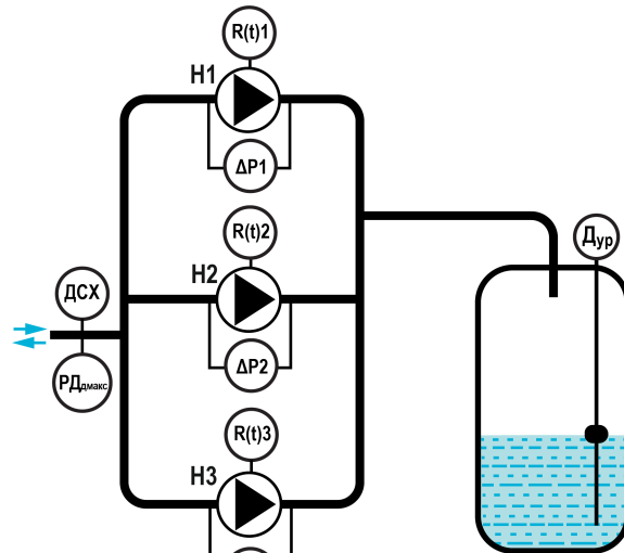
Рисунок 7.1 – Объект управления
