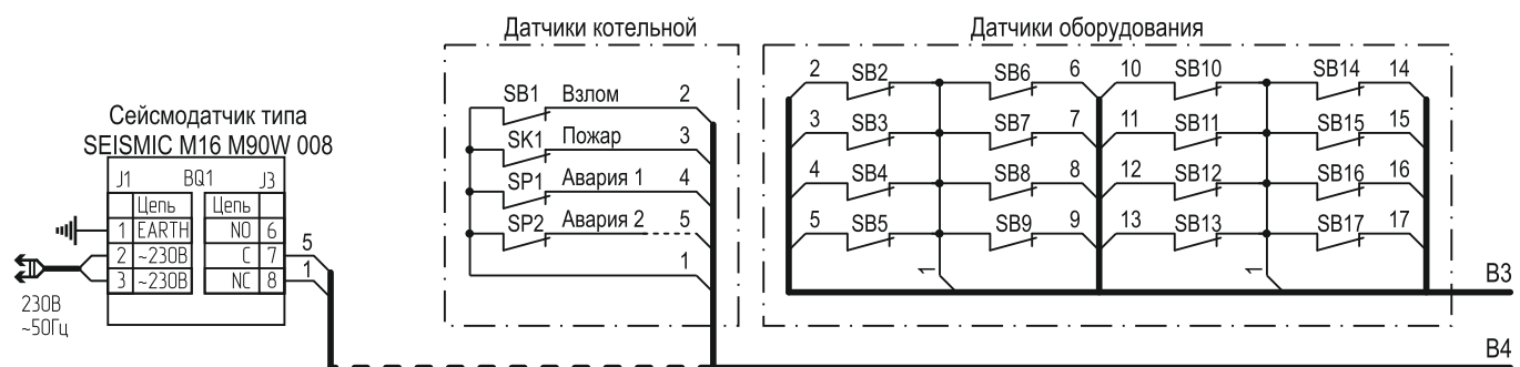
Схема подключения датчиков с нормально разомкнутыми контактами
