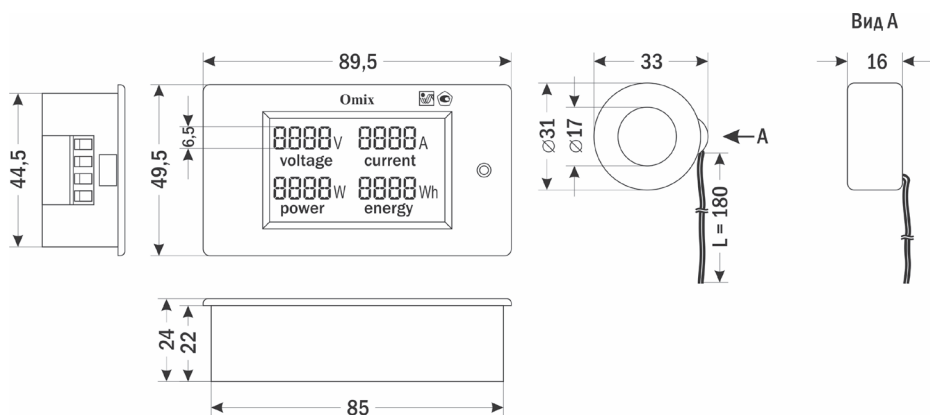
Рис. 3 – Размеры прибора
