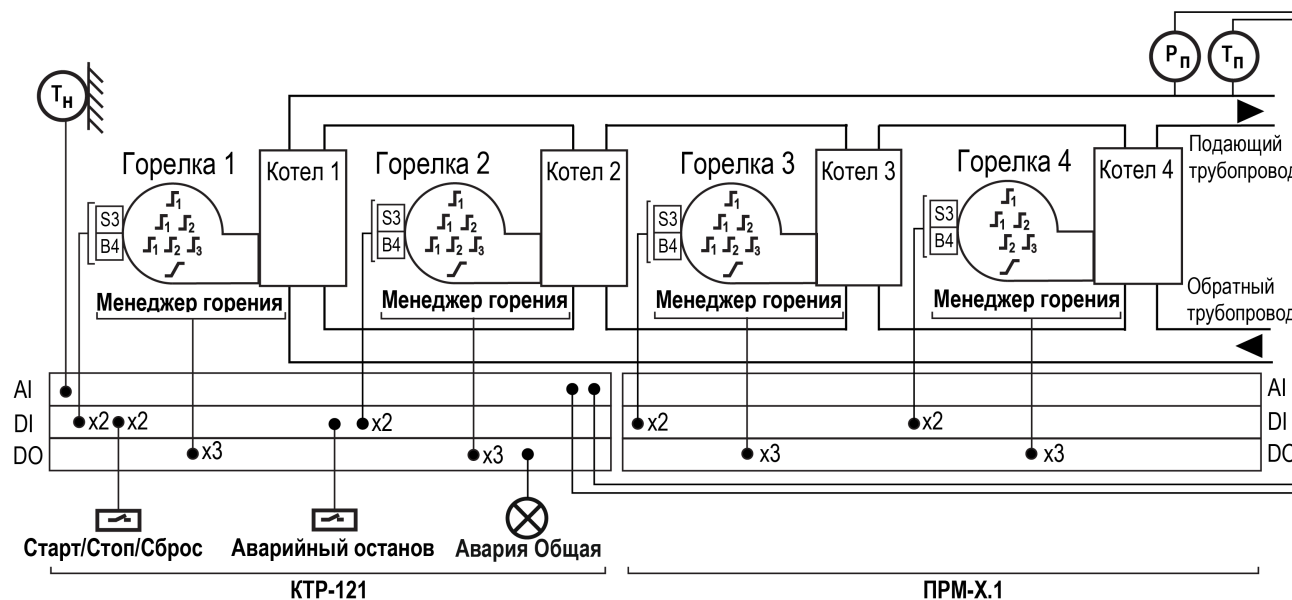
Рисунок 1.1 – Объект управления
