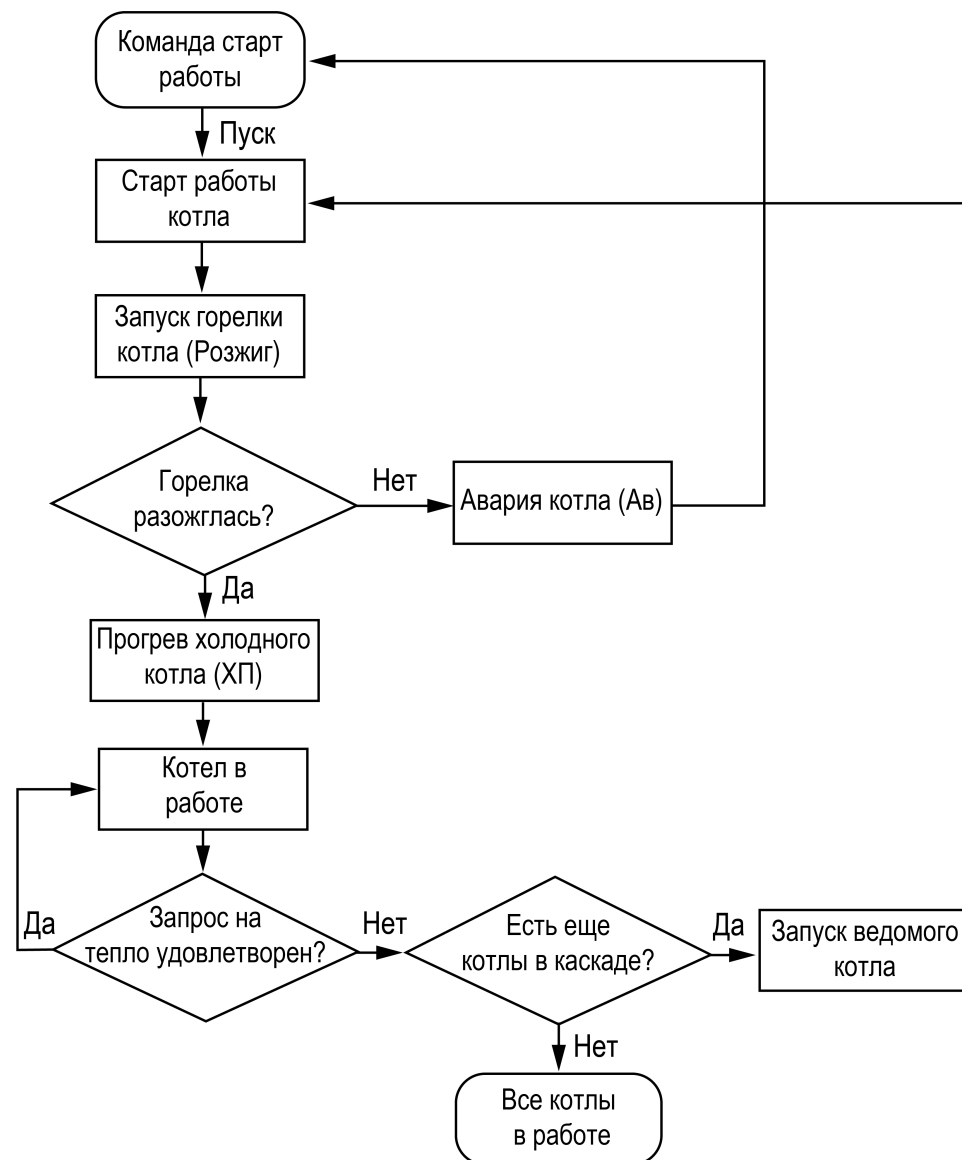
Рисунок 10.1 – Алгоритм запуска
