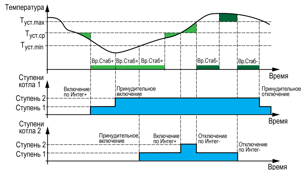
Рисунок 10.2 – Регулирование температуры
