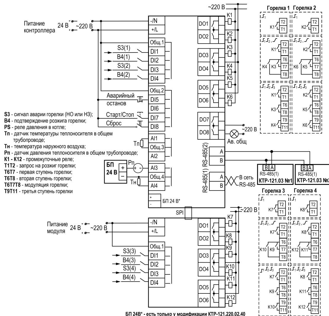
Рисунок 7.4 – Схема подключения КТП-121.02.40 и ПРМ-1 для управления котельной с четырьмя котлами и ГВС
