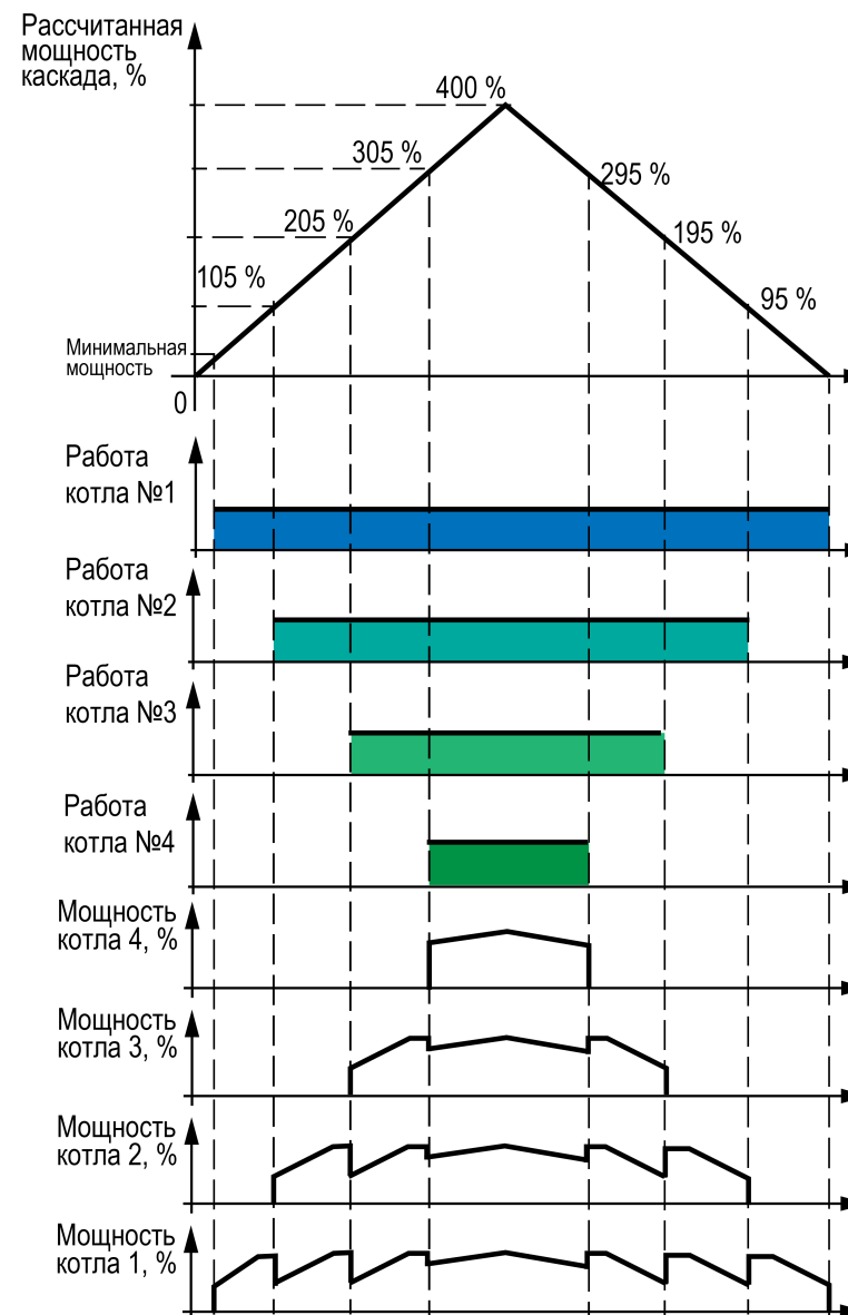
Рисунок 10.7 – Работа каскада котлов с модулируемыми горелками
