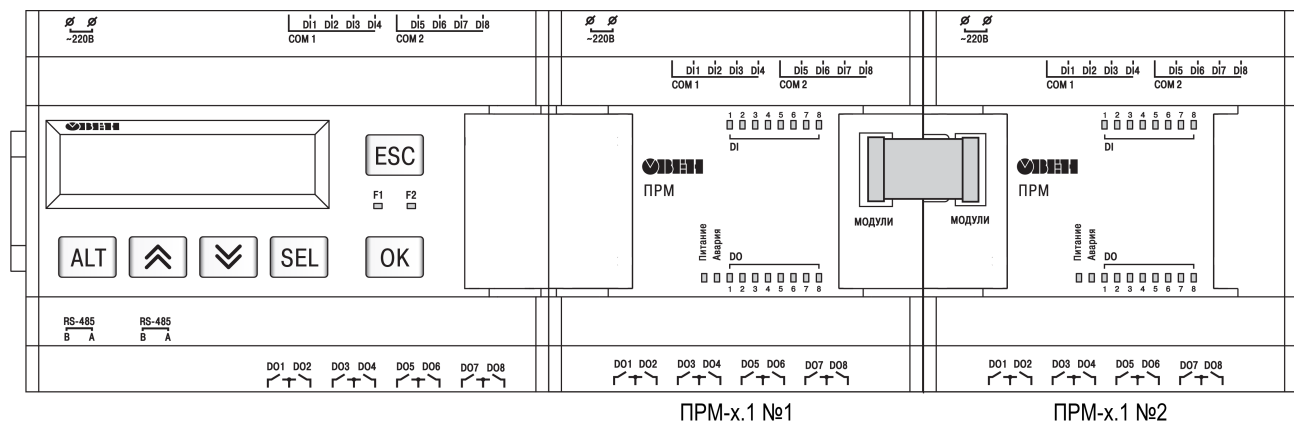
Рисунок 7.5 – Схема расположения модулей ПРМ-1
