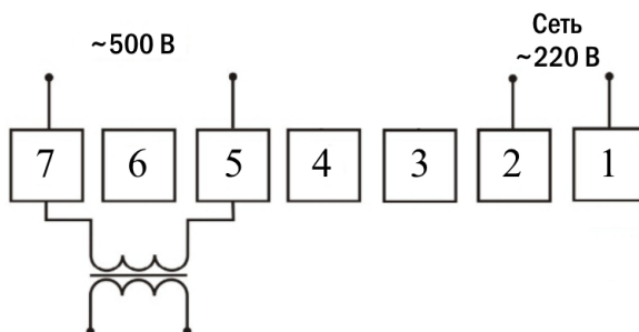
Рис. 9 – Схема подключения прибора. Тип корпуса P77
