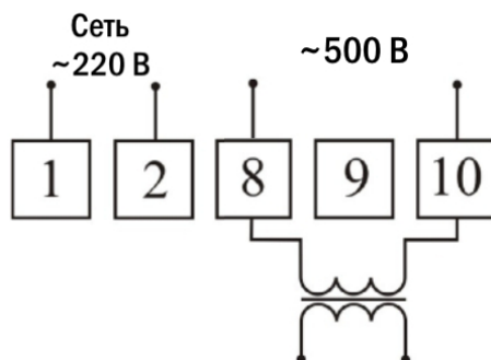
Рис. 10 – Схема подключения прибора. Типы корпусов: P94, P99, P1212
