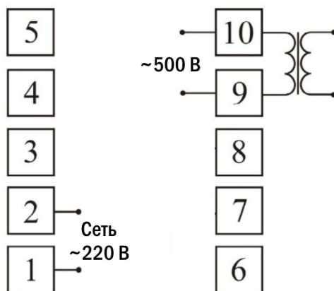
Рис. 8 – Схема подключения прибора. Тип корпуса P44
