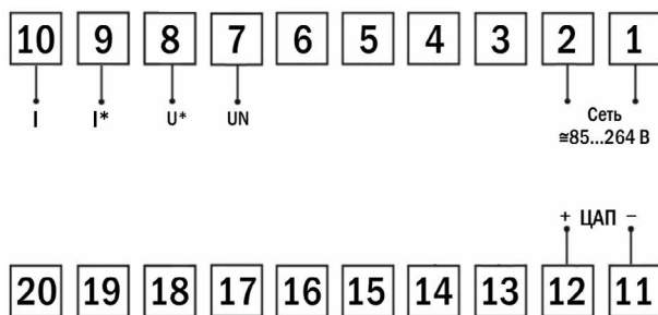
Рис. 7– Схема подключения прибора. Типы корпусов: P99, P1212
