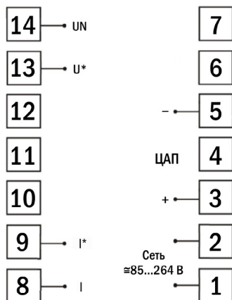
Рис. 6 – Схема подключения прибора. Тип корпуса P77
