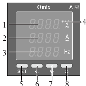
Рис. 1 – Управляющие элементы
