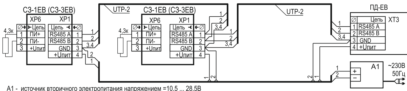
Типовая схема соединений с питанием от вторичного источника электропитания
