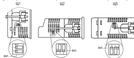
Рисунок 20 – Расположение DIP-переключателей
