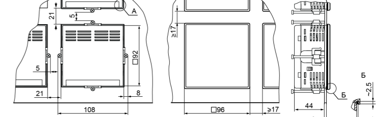
Рисунок 3 – Корпус Щ1 в щите толщиной 3 мм
