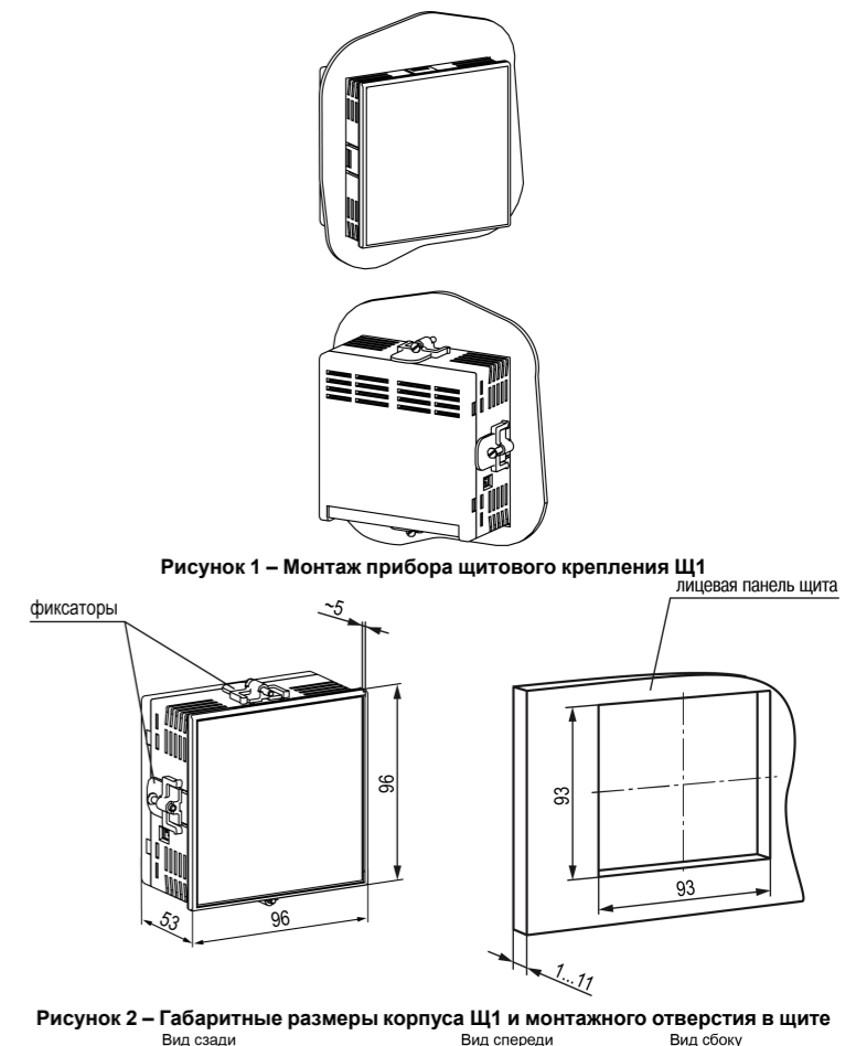
Рисунок 1 – Монтаж прибора щитового крепления Щ1
