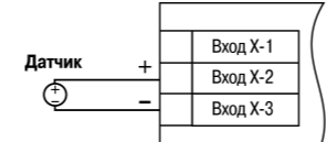
Рисунок 18 – Схема подключения активного датчика с выходом в виде напряжения -50...+50 мВ или 0...1 В
