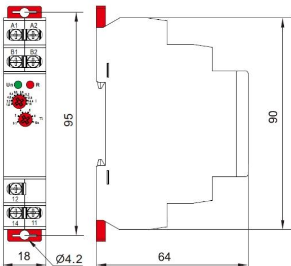
Рис. 3 – Размеры прибора
