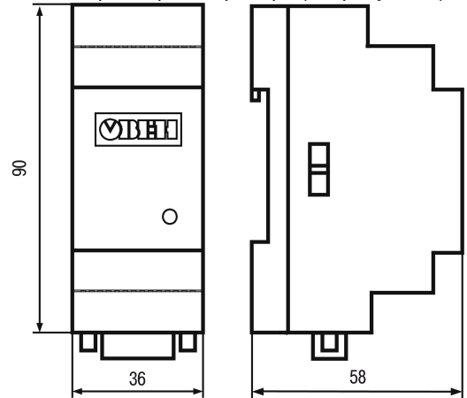
Рисунок 2 – Габаритные размеры прибора
